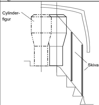
Mått: A = 300 mm, C = 450 mm, B = 300 mm, H = 1500 mm. Figur 2
