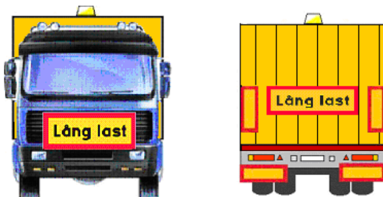
Figur 3 Varningsskyltar framåt och bakåt (2 kap. 5 §) och rektangulära skyltar (reflexanordningar) bakåt (2 kap. 6 §)
