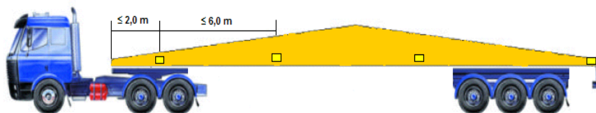
Figur 4 Sidomarkeringslyktor och sidomarkeringsreflexer på sidan på mellanliggande last och längst bak på sidan på utskjutande last (2 kap. 9 §)
